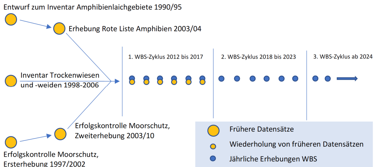
Ablauf und verwendete Datensätze der Wirkungskontrolle Biotopschutz Schweiz WBS
