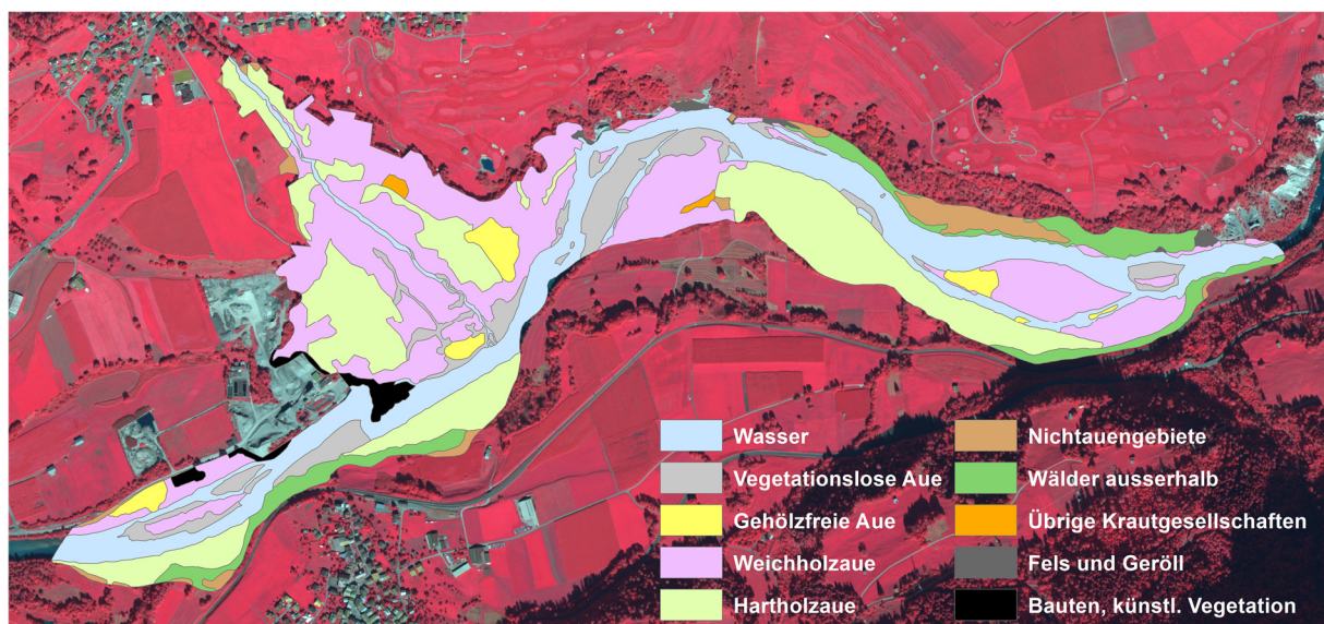
Kartierung der Deltas, Seeufer und Flussauen nach Formationen mittels eines Farbinfrarot-Luftbilds (am Beispiel einer Flussau).
